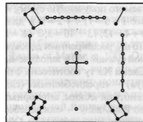
Рис. 2а. Древнее изображение схемы Ло шу
